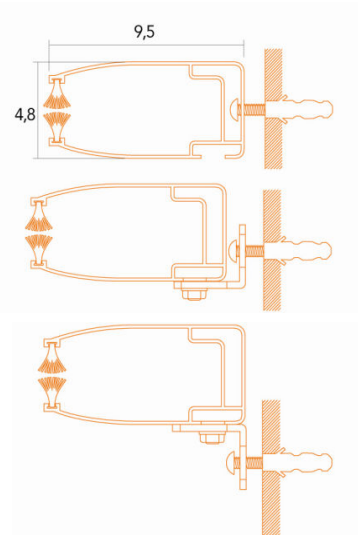
βάση & τρόποι στήριξης guide support & fixing ways
