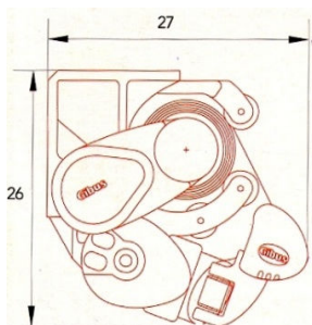
χωρίς σκέπαστρο / no cover
