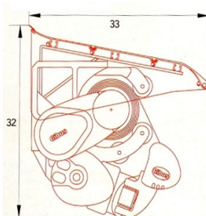
με σκέπαστρο / with cover
