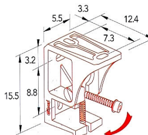
ζάση τοίχου - μαρκίζας / wall-roof support
