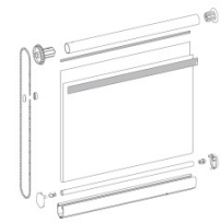
μηχανισμός διπλού ρόλλερ DTL double roller mechanism DTL
